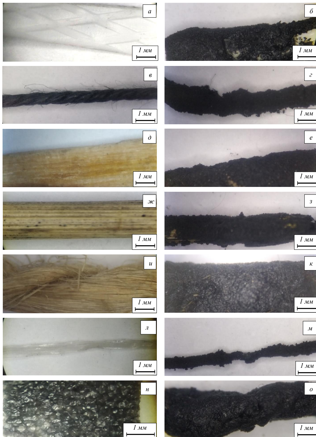
Рис. 3. Внешний вид ПА (а, в, д, ж, и, л, н) и СА (б, г, е, з, к, м, о) Fig. 3. Appearance of pore-forming additives (а, в, д, ж, и, л, н) and structural aggregates (б, г, е, з, к, м, о)
