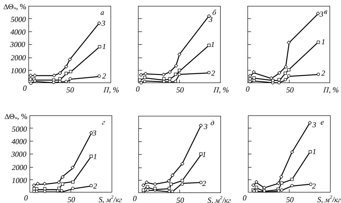
Рис. 4. Зависимость прироста массы ЖС (1), ОММ (2), ЖК (3) от пористости и удельной поверхности порообразующих добавок при температуре t_{OMM} 20 (а, г), 50 (б, д) и 90 °С (в, е)
