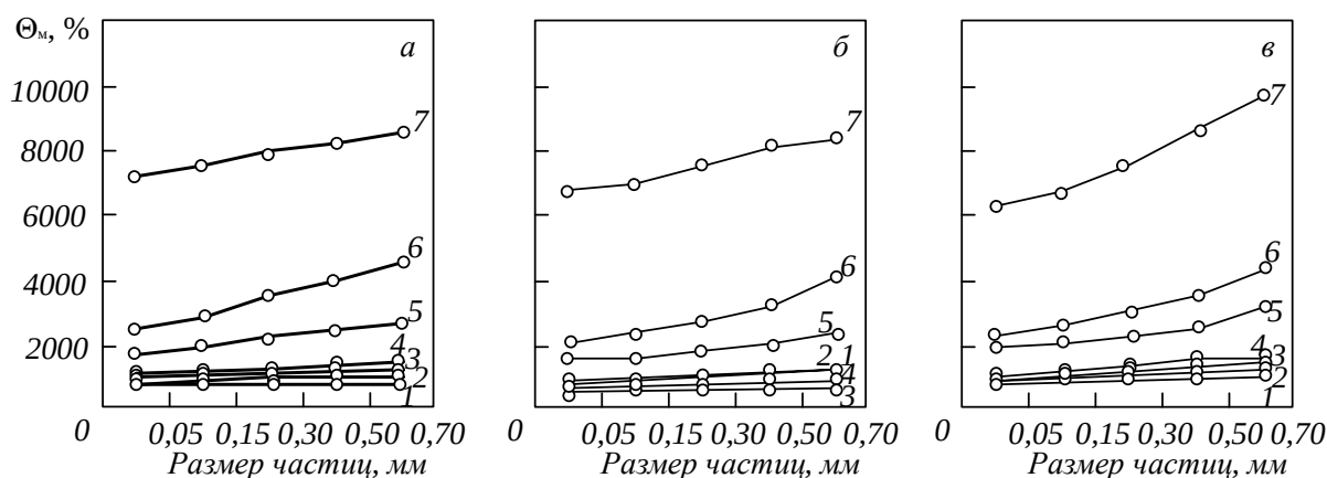
Рис. 5. Зависимость относительной массы СА от размера частиц железорудного концентрата (а), угольной (б) и известковой (в) добавок и от типа ПД при температуре t_{OMM} = 20 °С (цифры у кривых соответствуют нумерации в табл. 1.)
