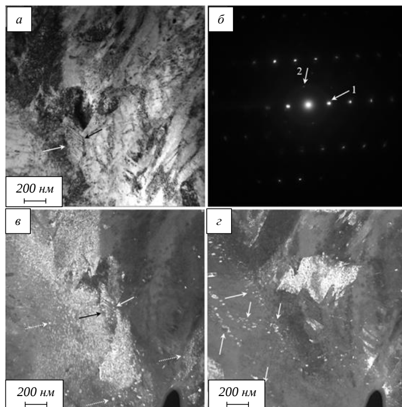
Рис. 2. Электронно-микроскопическое изображение структуры переходной зоны после наплавки (исходное состояние): а – светлое поле; б – микроэлектроннограмма; в и г – темные поля, полученные в рефлексах [110]\alpha\text{-Fe} + [002]\gamma\text{-Fe} + [012]\text{V}_2\text{C} и [110]\alpha\text{-Fe} + [103]\text{MoC} + [101]\text{W}_2\text{C} ; 1 и 2 – рефлексы, в которых получены темные поля для поз. в и г Fig. 2. Electron microscopic image of the structure of the transition zone in the state after surfacing (initial state): а – light field; б – microelectronogram; в and г – dark fields obtained in reflexes [110]\alpha\text{-Fe} + [002]\gamma\text{-Fe} + [012]\text{V}_2\text{C} and [110]\alpha\text{-Fe} + [103]\text{MoC} + [101]\text{W}_2\text{C} ; 1 and 2 – are reflexes in which dark fields are obtained for pos. в and г
