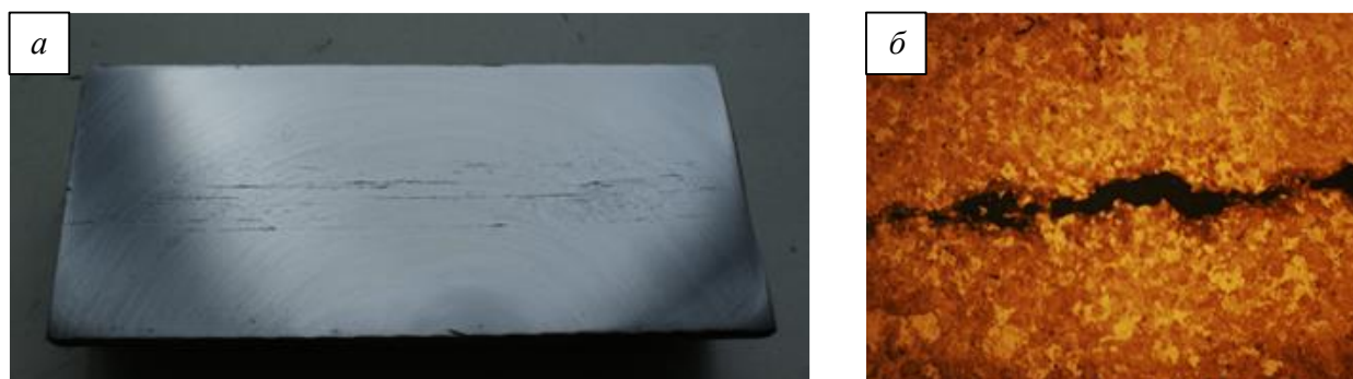
Рис. 3. Флокены в продольных образцах заготовок: а – шлифованные образцы; б – образцы после травления Fig. 3. Floccules in longitudinal samples of workpieces: a – ground samples; b – samples after etching
